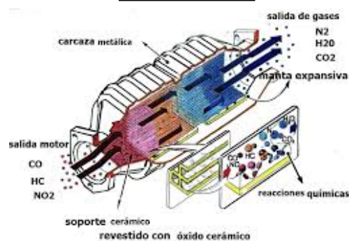
1 corte de un convertidor catalítico
