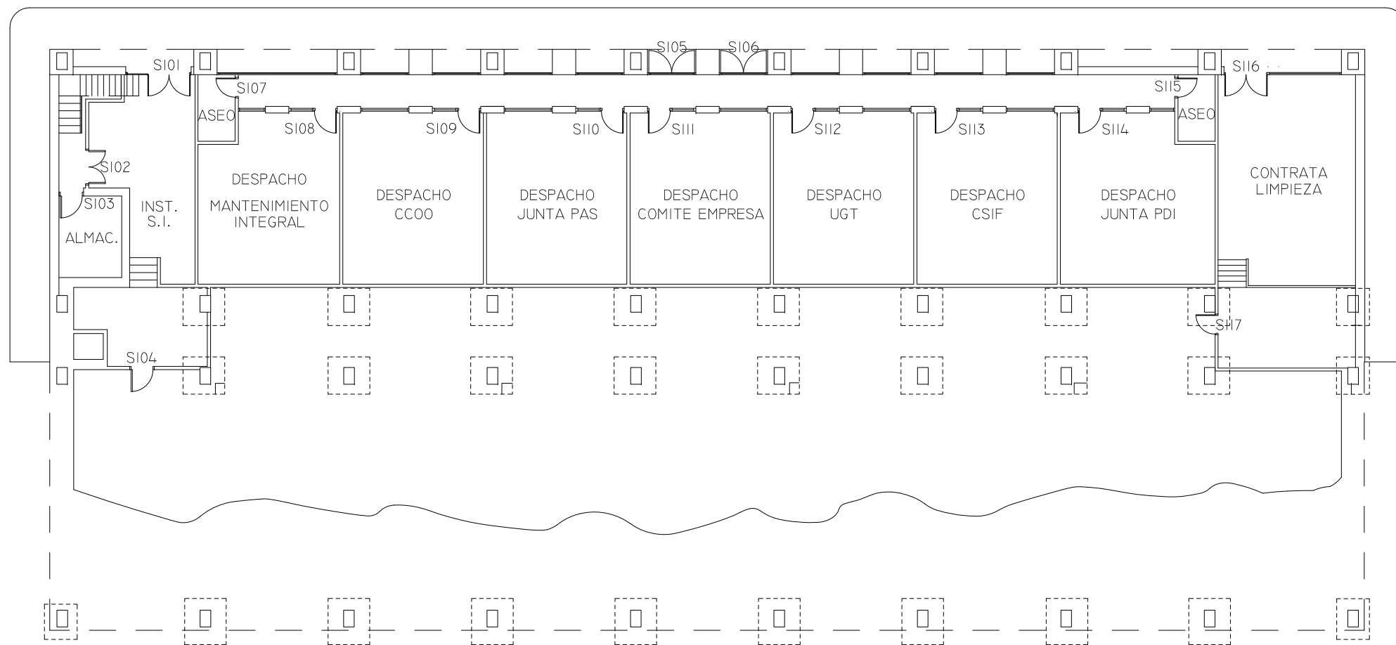
PLANTA SOTANO
